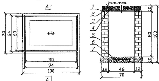
ДЕТАЙЛ - ШАХТА 60/90
